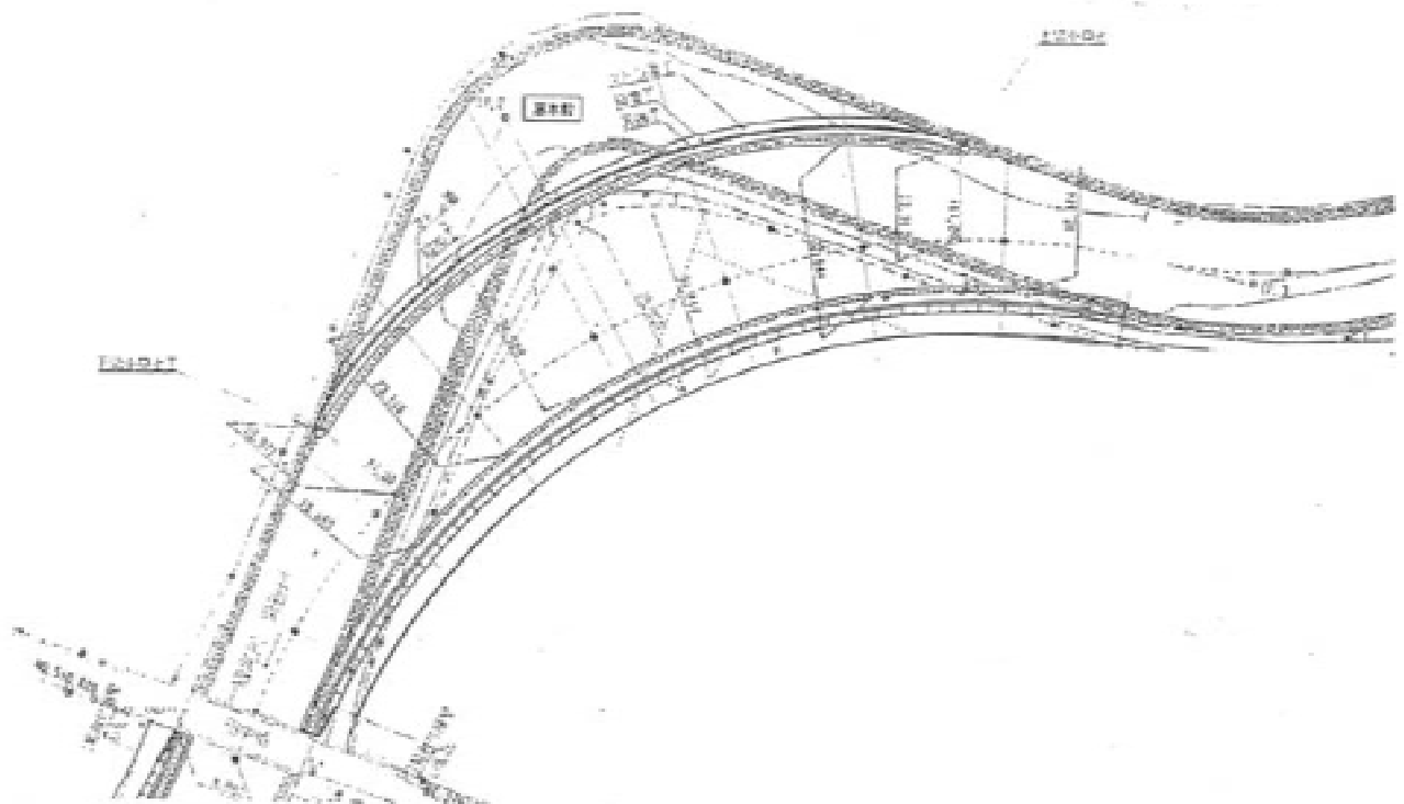
平面図（湾曲改修部）
